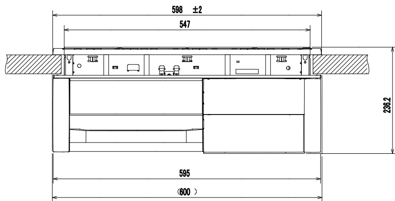
【正面図】
